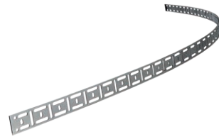
Rugalmas sín, hossza 185cm, 1 darab Minimális ívsugár: 1,0 m PRW-0466-50-01-01-0
