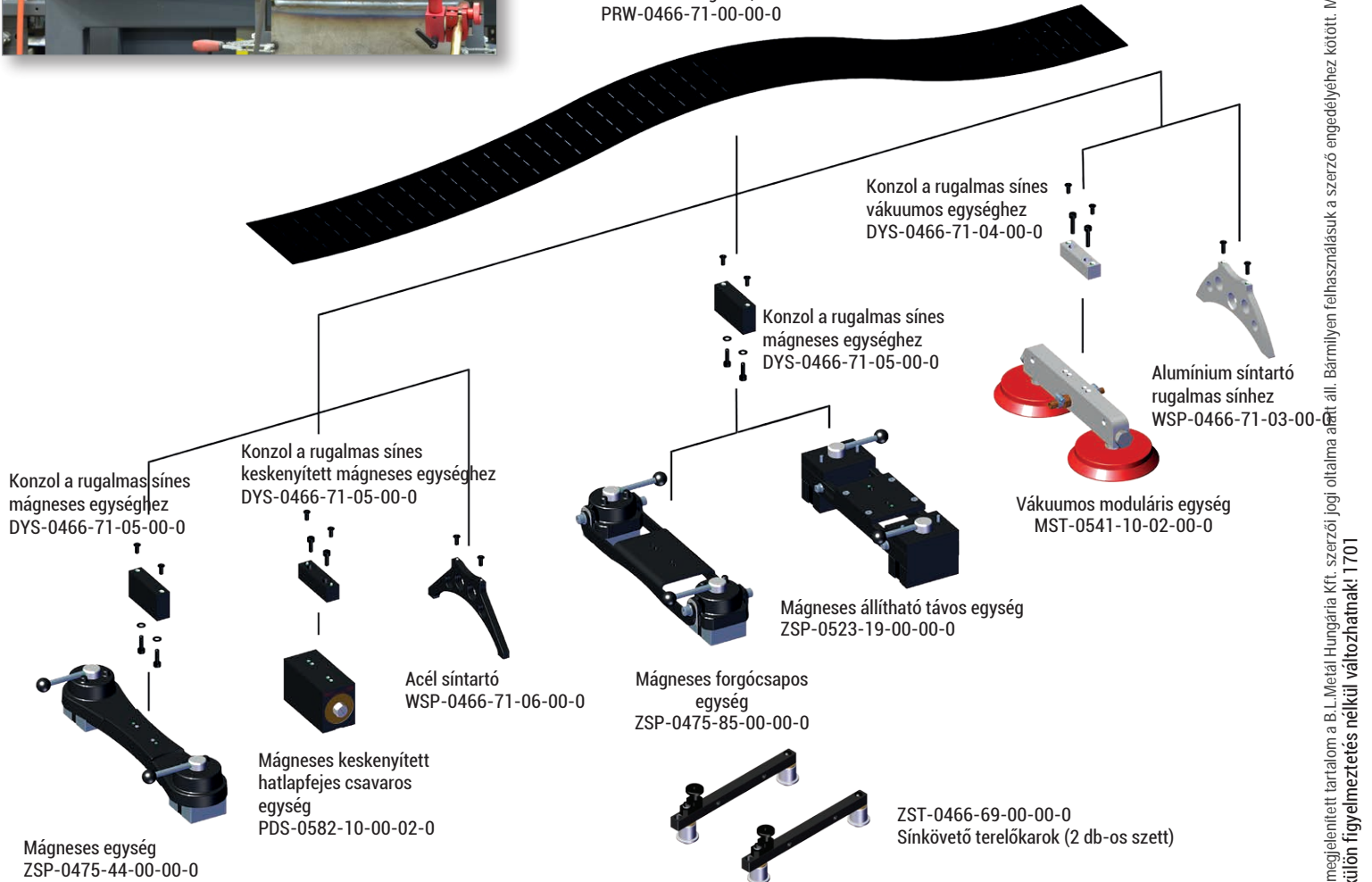
Merevített pálya, hossza 1,88 m Minimális ívsugár: 1,25 m PRW-0466-71-00-00-0
